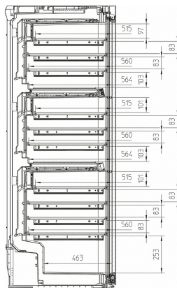
KWT6831SG, KWT6832SGS, KWT6833SG, KWT6834SGS (asennuspiirustukset)
