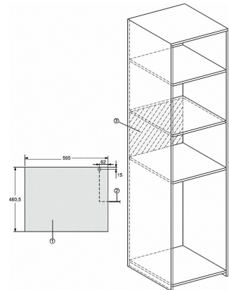
M2240SC, asennuspiirustukset
