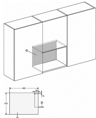
M2224SC, asennuspiirustukset
